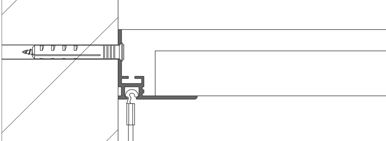
STAS systeemplafond rail Afmetingen 31 x 35 mm
