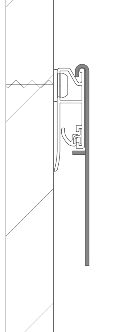
STAS papergriphanger Afmetingen 3,5 x 9,5 mm
